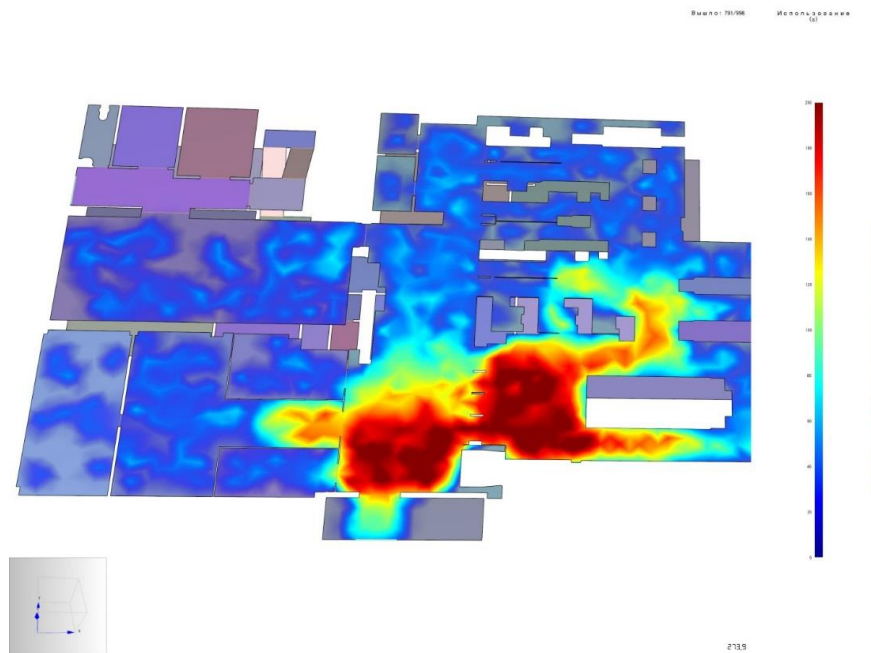
Рис. 9. Графічне зображення щільності людського потоку
