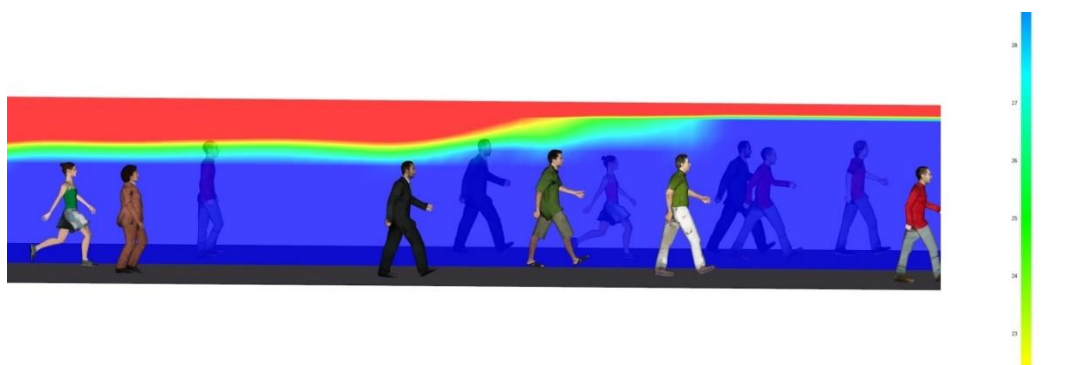
Рис. 8. Ілюстрування поширення небезпечних факторів пожежі
